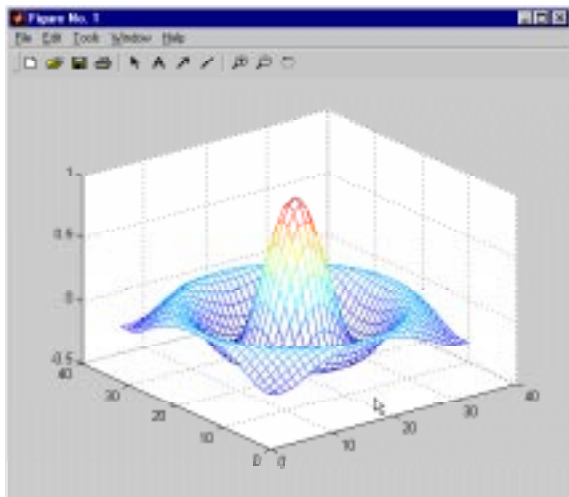
Figura 18. Figura 3D de la función “sombrero”.
