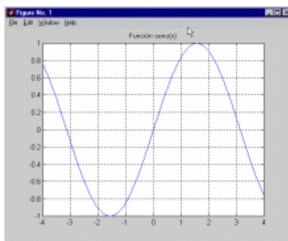
Figura 2. Gráfico de la función \text{seno}(x) .
