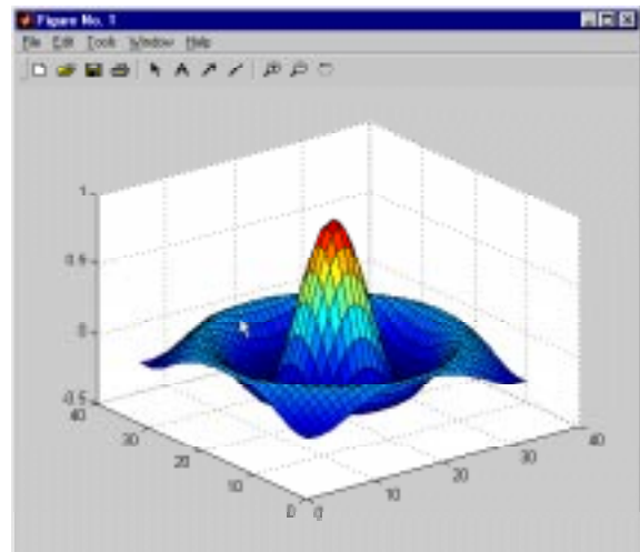
Figura 19. Función “sombrero” con facetas.
