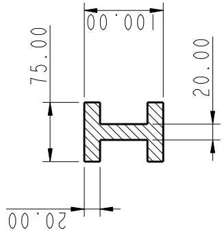
Seccion AA
